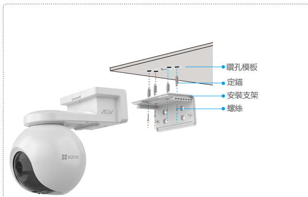
圖 1 天花板安裝
