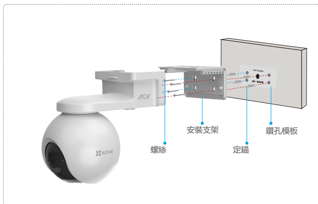
圖 2 壁掛式安裝
